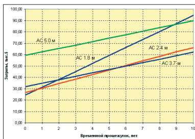
Рис. 5. Суммарные затраты на радиолинию для ЭИИМ=44,7 дБВт
